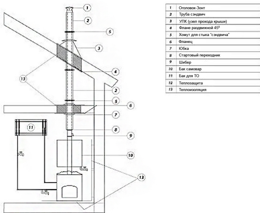
Рис.3 Пример установки дымохода для банной печи
