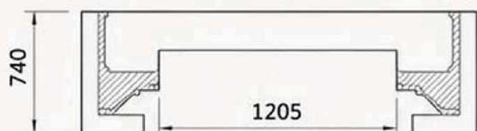
ВИД СВЕРХУ (РАЗРЕЗ)
