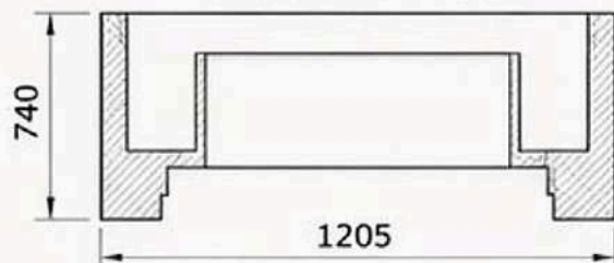
ВИД СВЕРХУ (РАЗРЕЗ)
