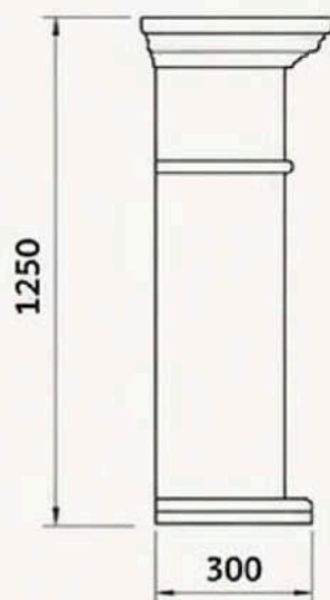
ВИД СБОКУ
