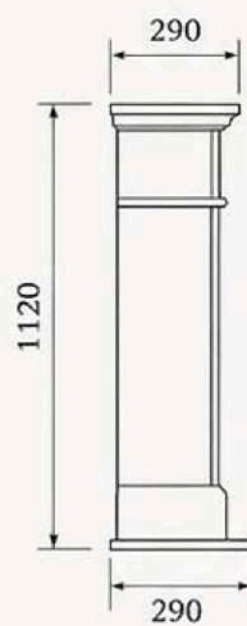
ВИД СБОКУ
