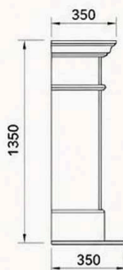
ВИД СБОКУ
