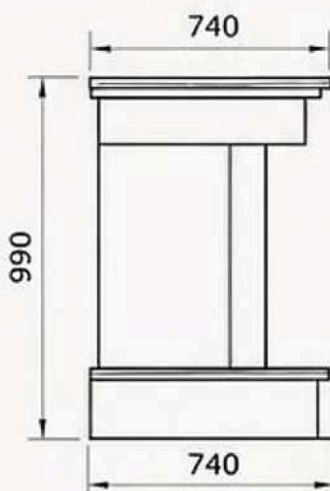
ВИД СБОКУ
