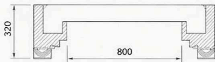
ВИД СВЕРХУ (РАЗРЕЗ)
