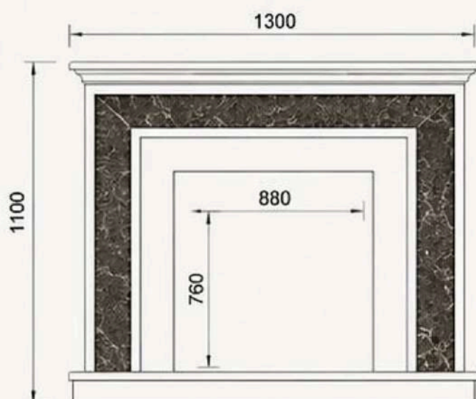
ВИД СПЕРЕДИ
