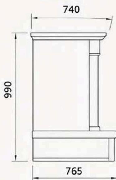
ВИД СБОКУ
