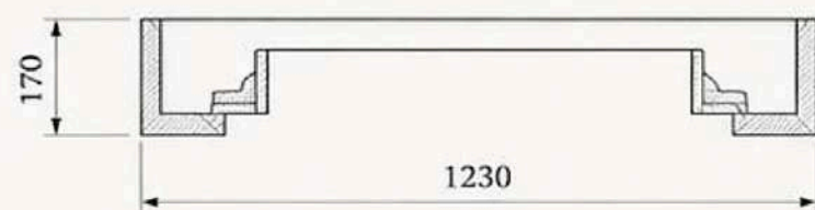
ВИД СВЕРХУ (РАЗРЕЗ)
