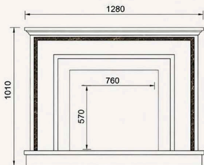
ВИД СПЕРЕДИ
