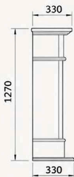
ВИД СБОКУ
