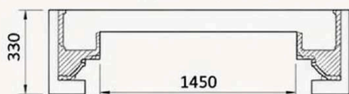
ВИД СВЕРХУ (РАЗРЕЗ)
