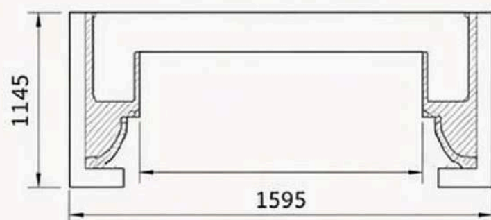
ВИД СВЕРХУ (РАЗРЕЗ)
