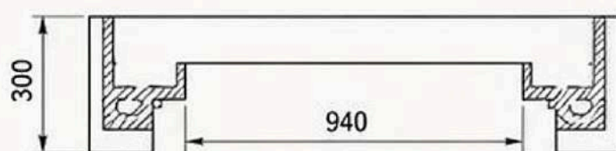
ВИД СВЕРХУ (РАЗРЕЗ)
