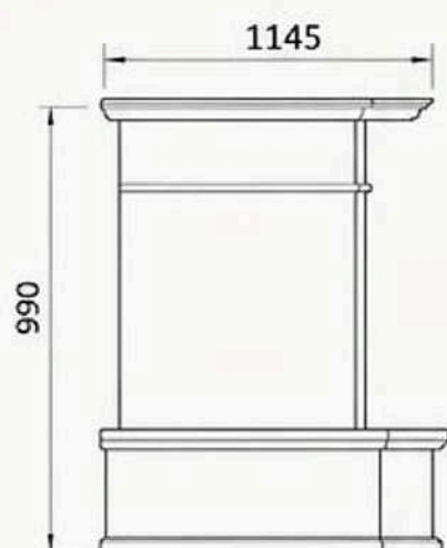
ВИД СБОКУ
