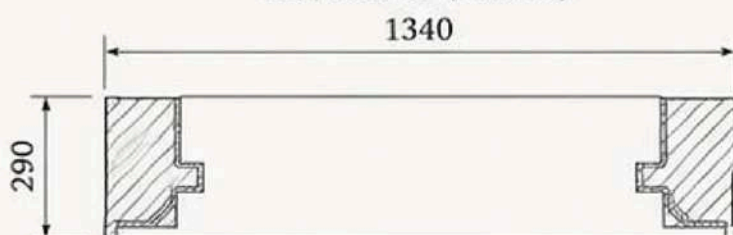
ВИД СВЕРХУ (РАЗРЕЗ)
