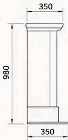
ВИД СБОКУ
