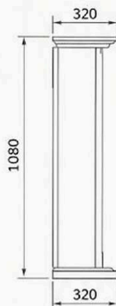
ВИД СБОКУ
