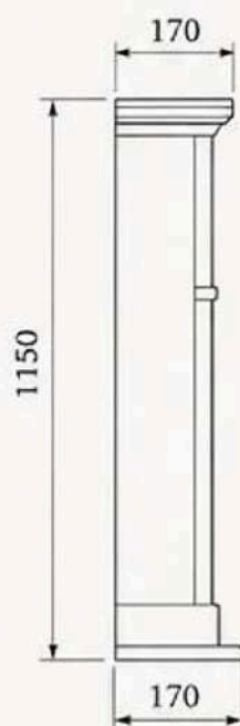
ВИД СБОКУ
