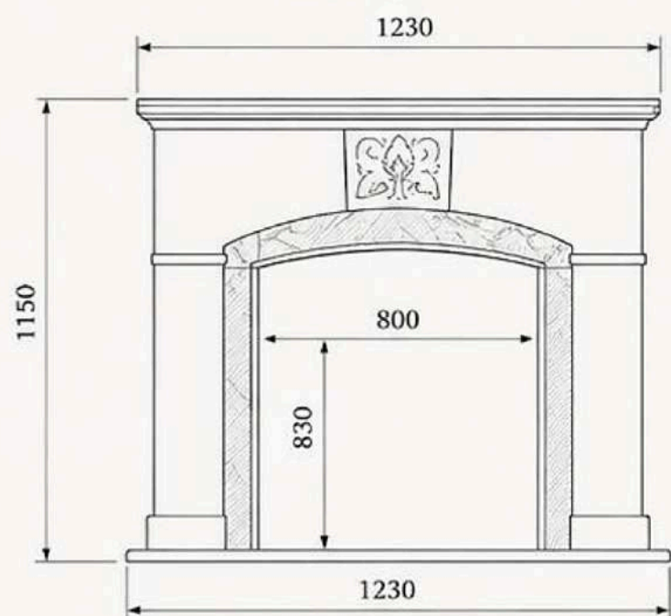
ВИД СПЕРЕДИ
