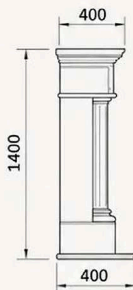
ВИД СБОКУ
